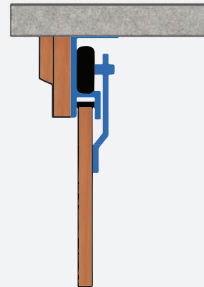
Sturzblende wenn kein Sturz vorhan- den
